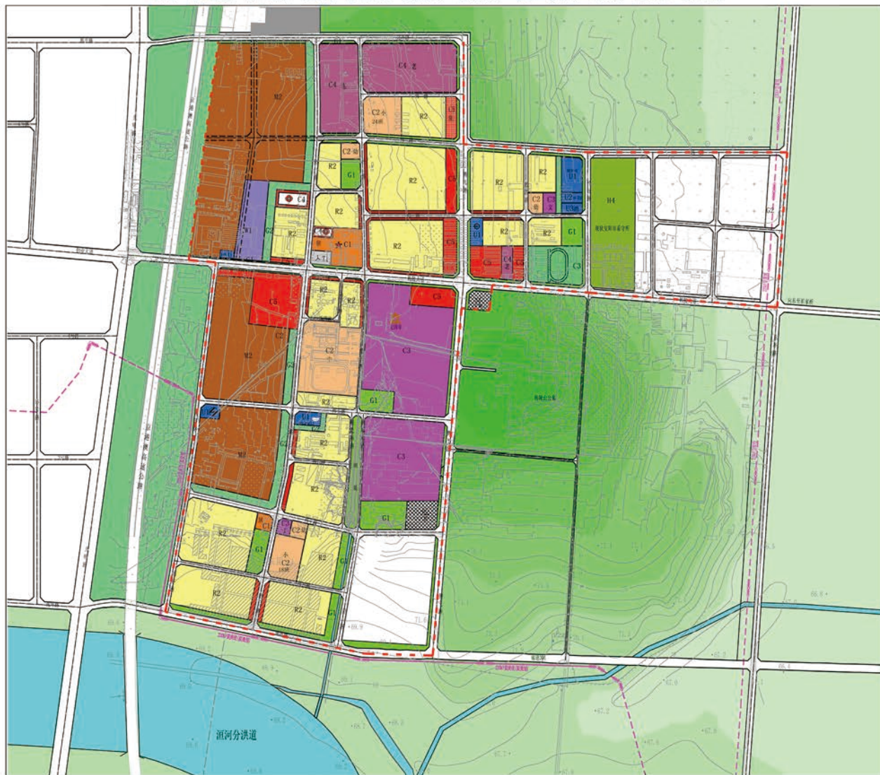
镇区用地规划图
