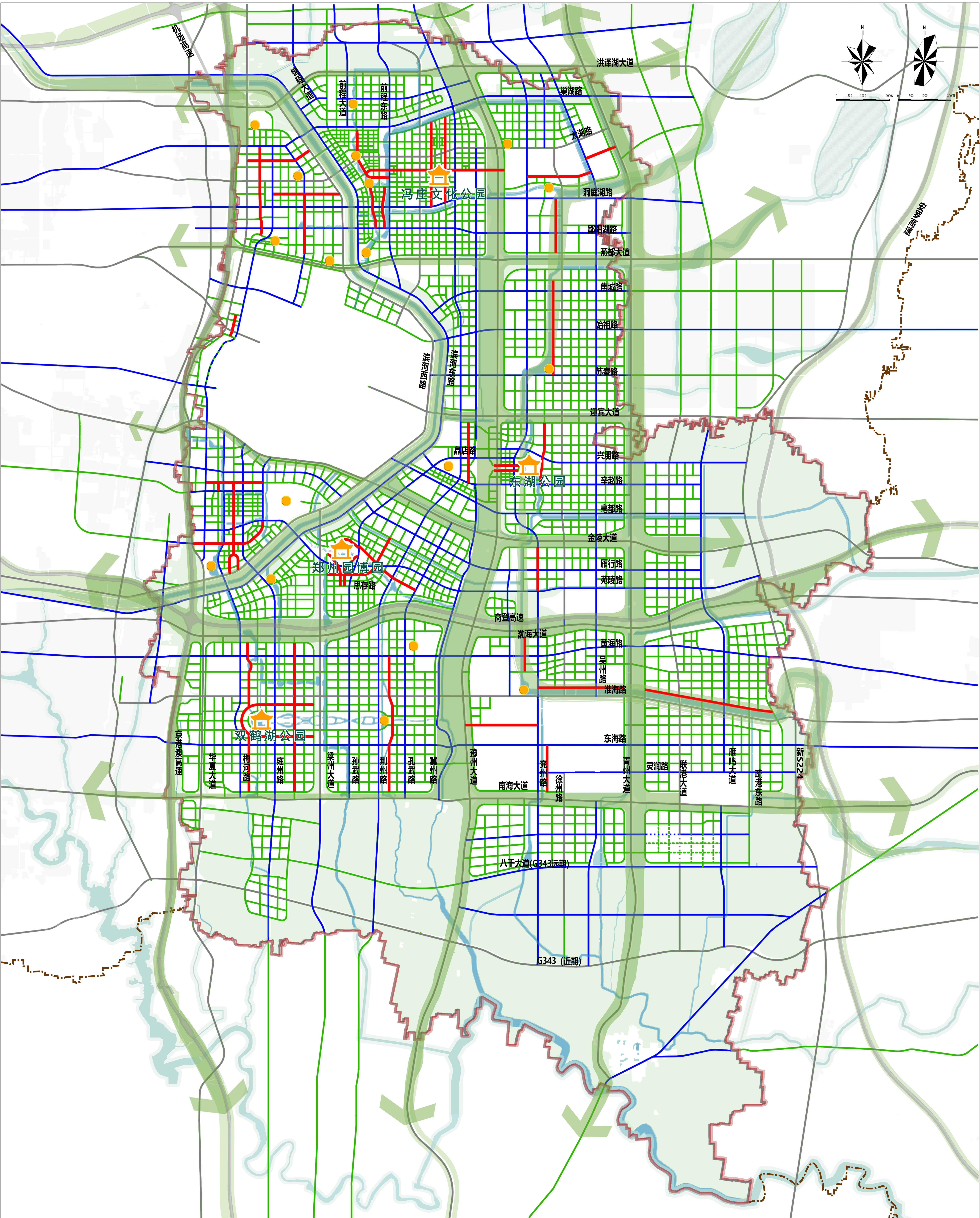
航空港区自行车、步行系统规划图
