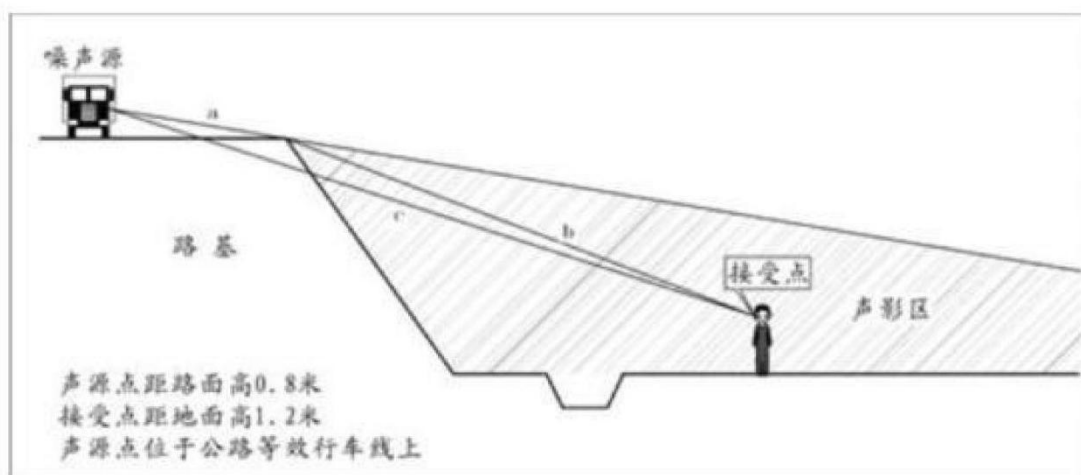
图10-4 声程差δ计算示意图
