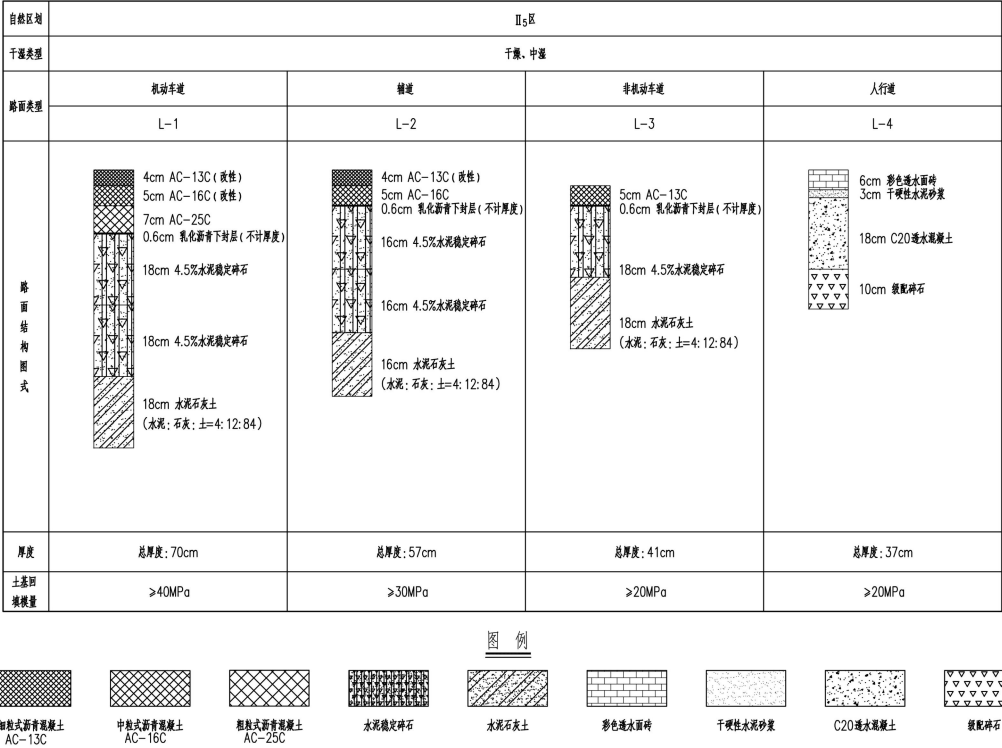
图 2 灵润路路面结构示意图
