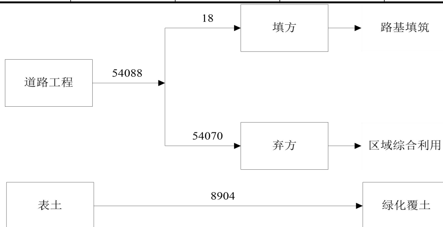
图3 土石方平衡图 (m 3 )
