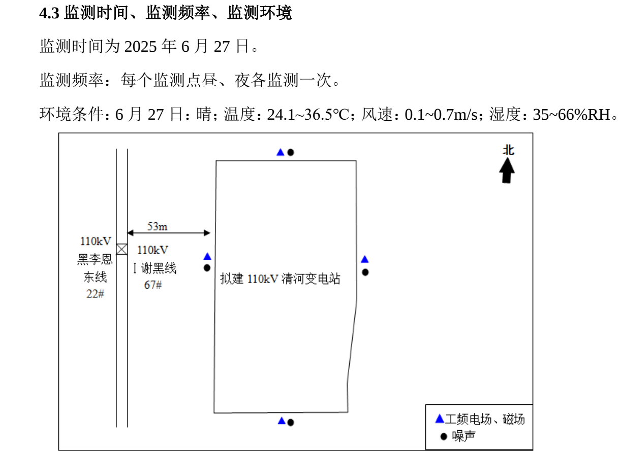
图 3-2 环境现状监测布点示意图
