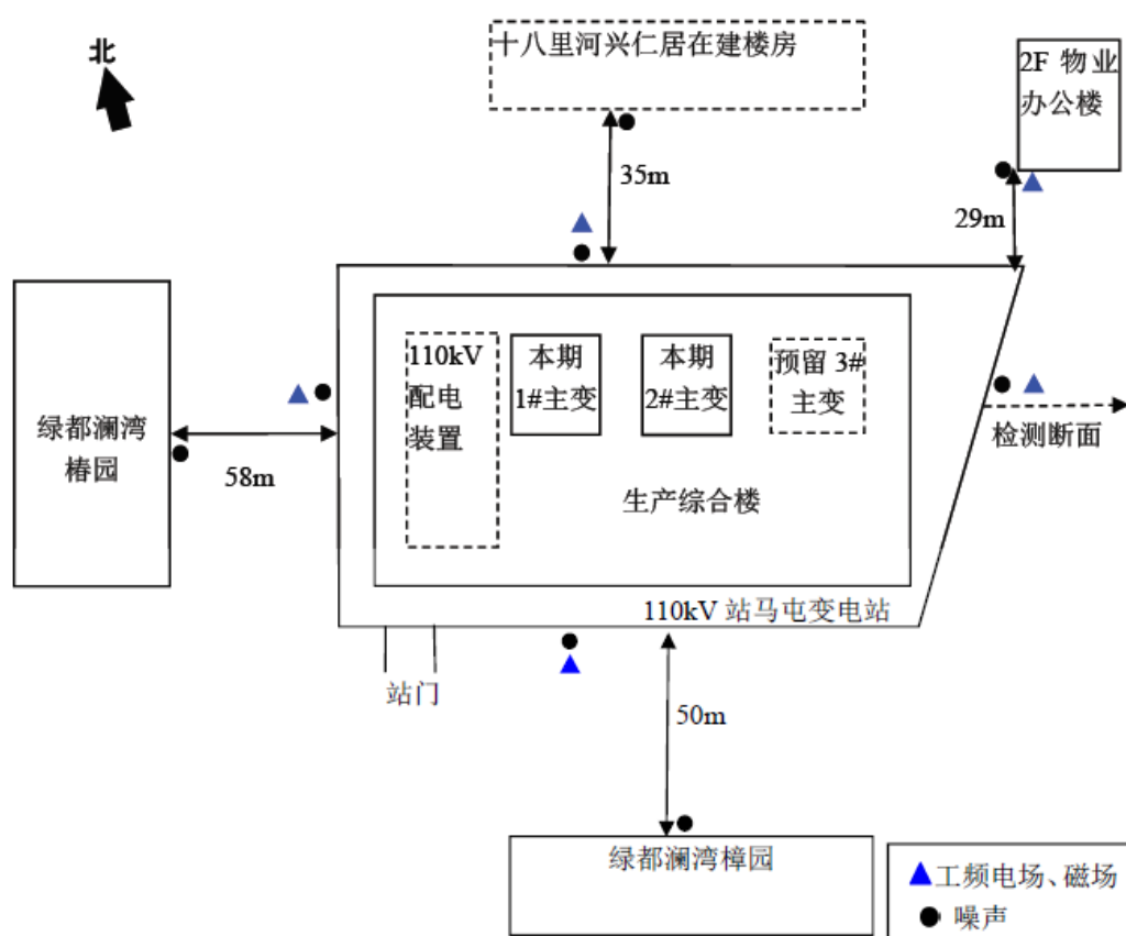
图 3-2 110kV 站马屯变电站类比监测布点图
