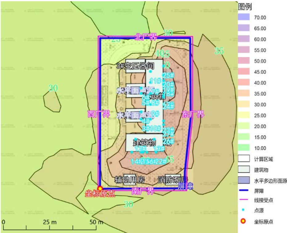
图 4-5 距离地面 1.2m 的噪声预测分布图
