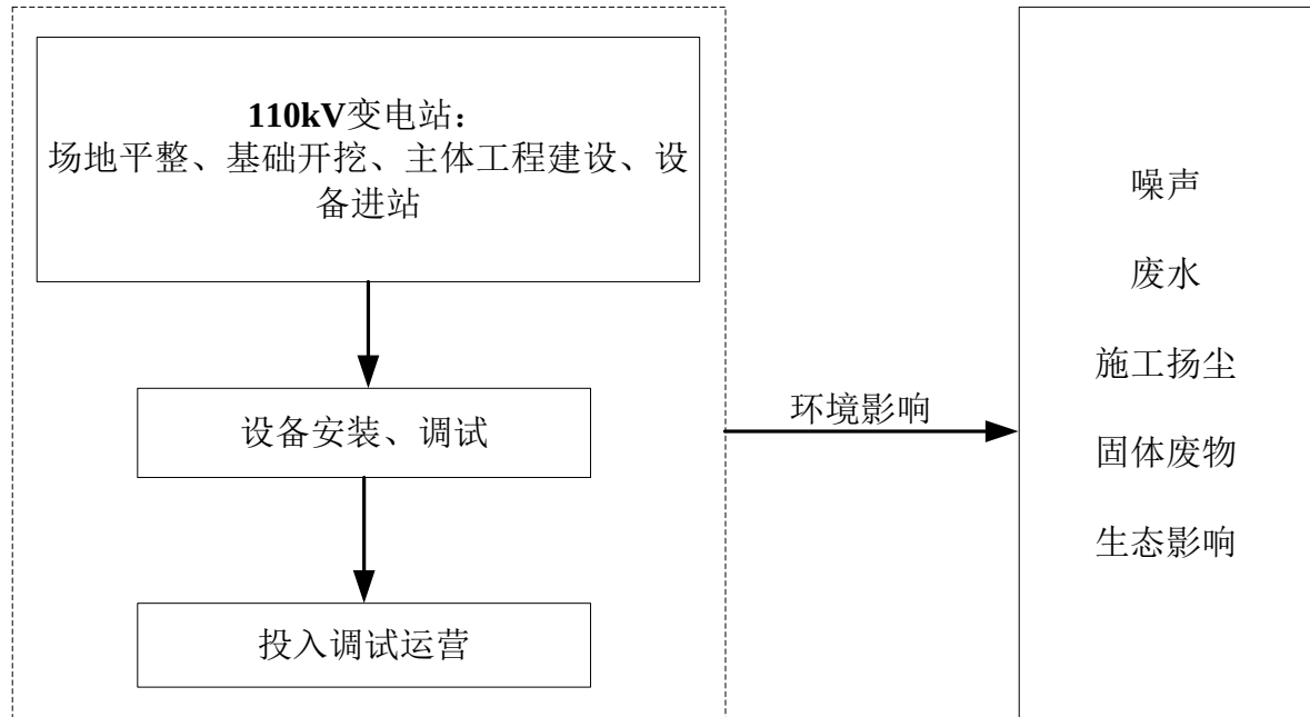
图 4-1 变电站施工期主要产污环节示意图
