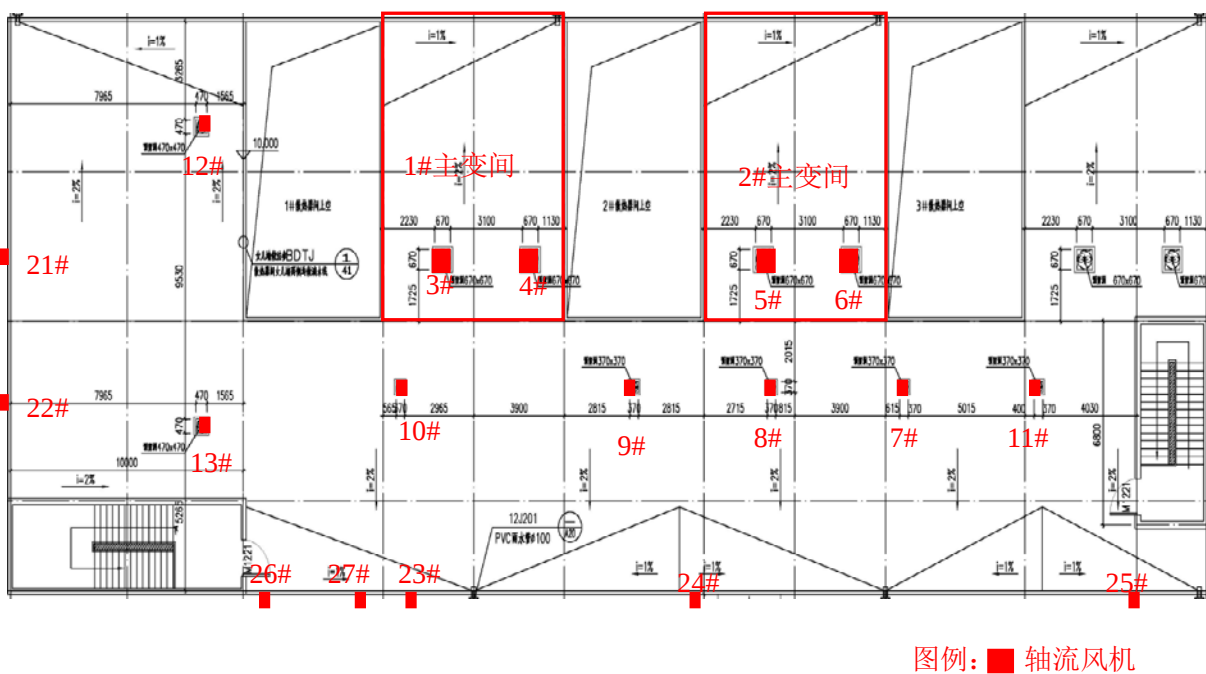
图 4-3 变电站声源分布情况示意图
