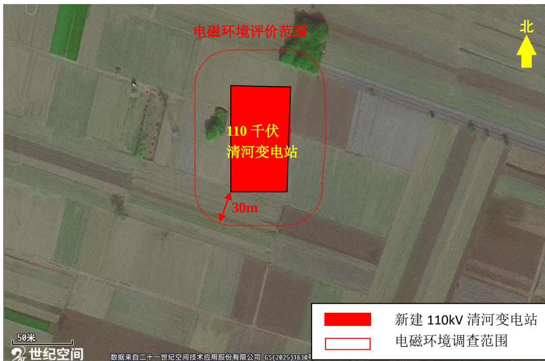
图 1-1 本工程电磁评价范围图
