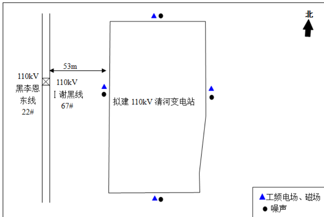
图 2-1 拟建 110kV 清河变电站四周厂界检测示意图
