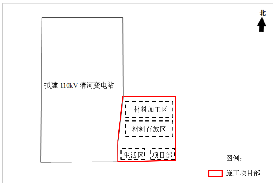
图 2-3 施工现场布置图
