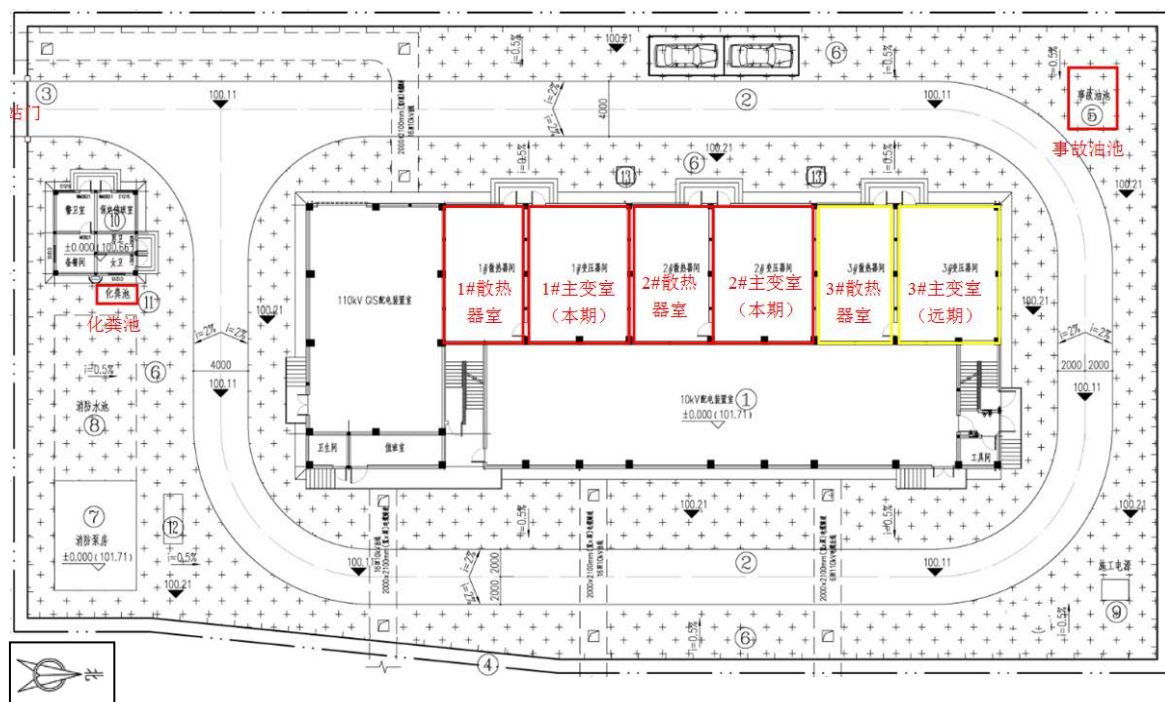
图 2-2 项目变电站平面布置图
