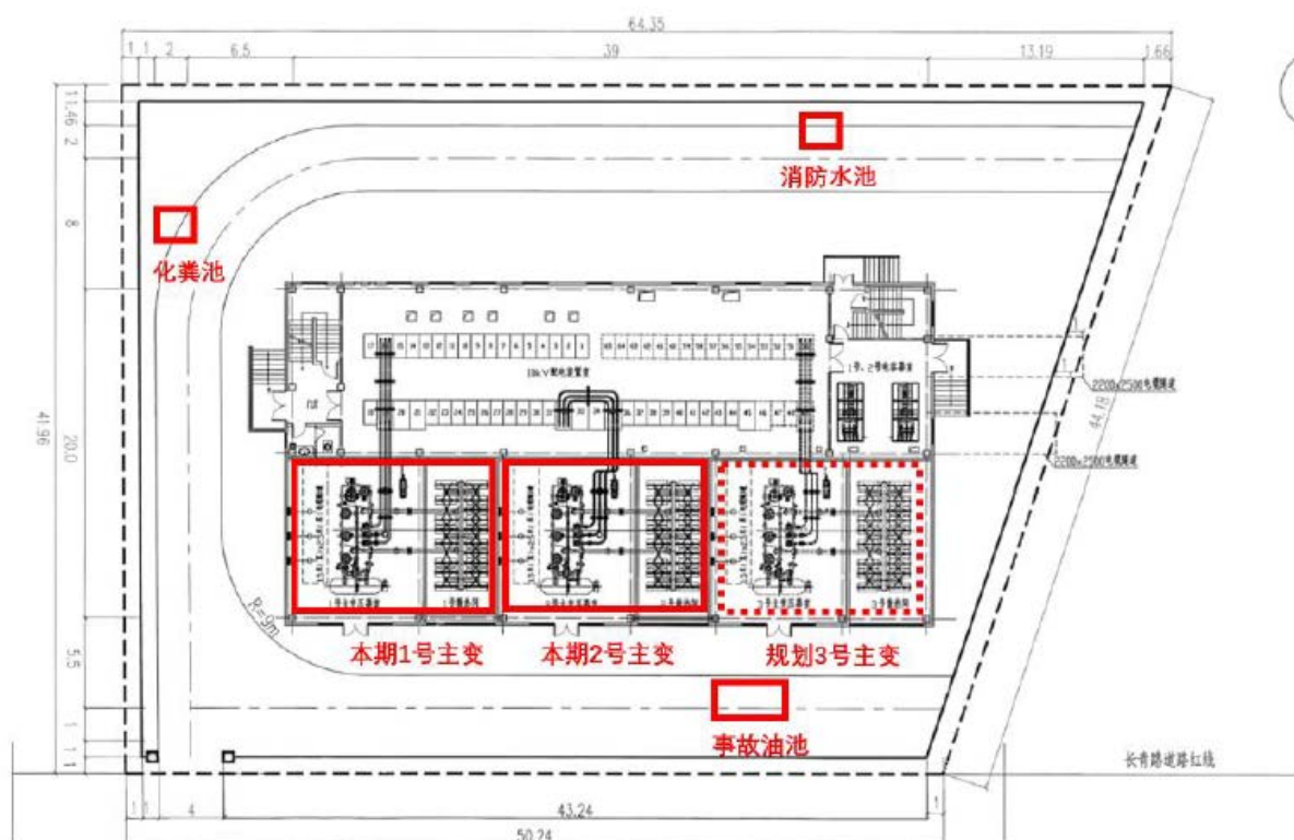
图 3-1 110kV 站马屯变电站平面布置图
