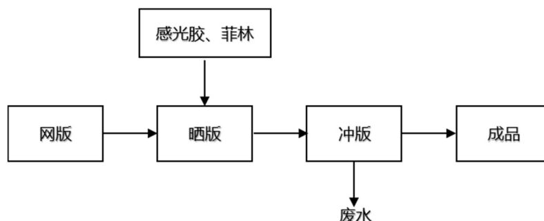
图5. 晒版工艺流程
