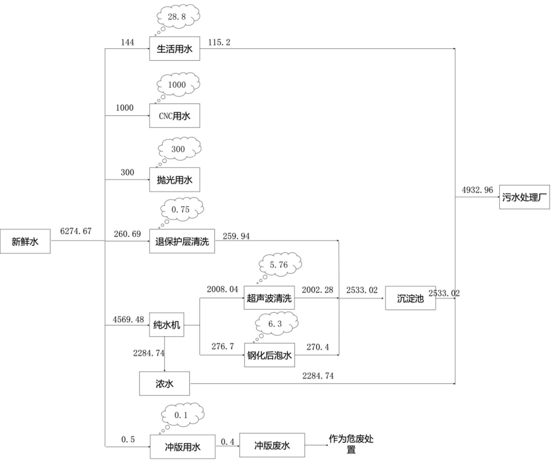
图1. 本项目水平衡图 (t/a)
