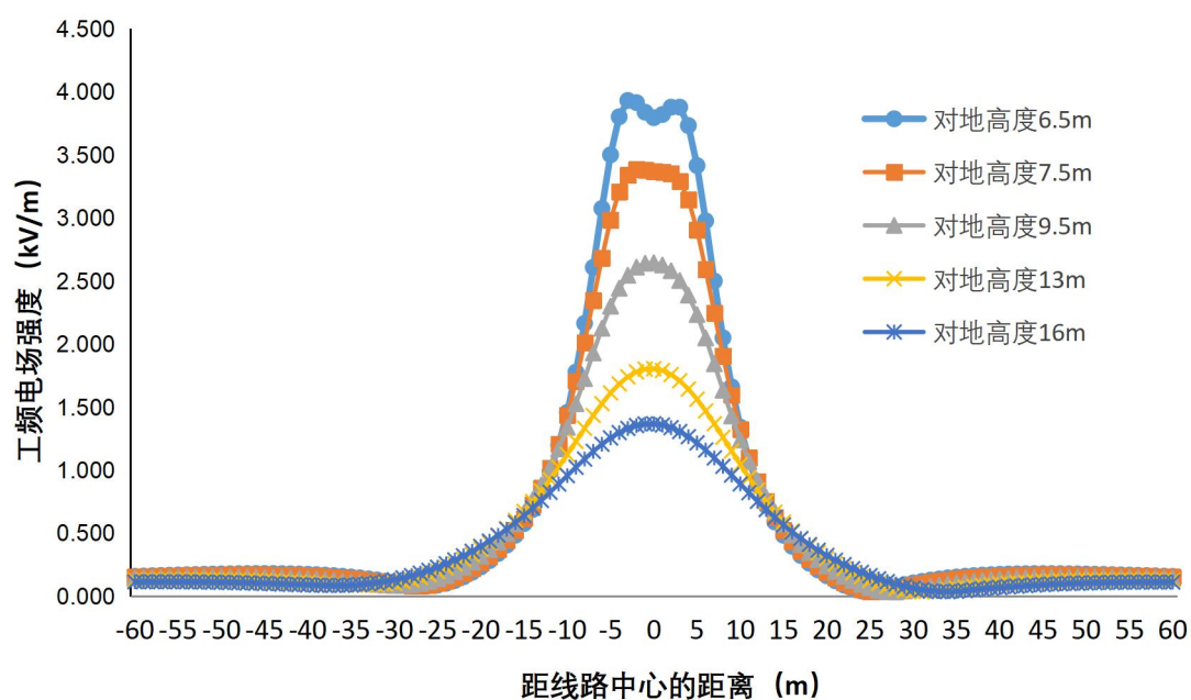
图 3-1 本工程本工程 110/220kV 混压同塔四回架空线路工频电场强分布趋势图
