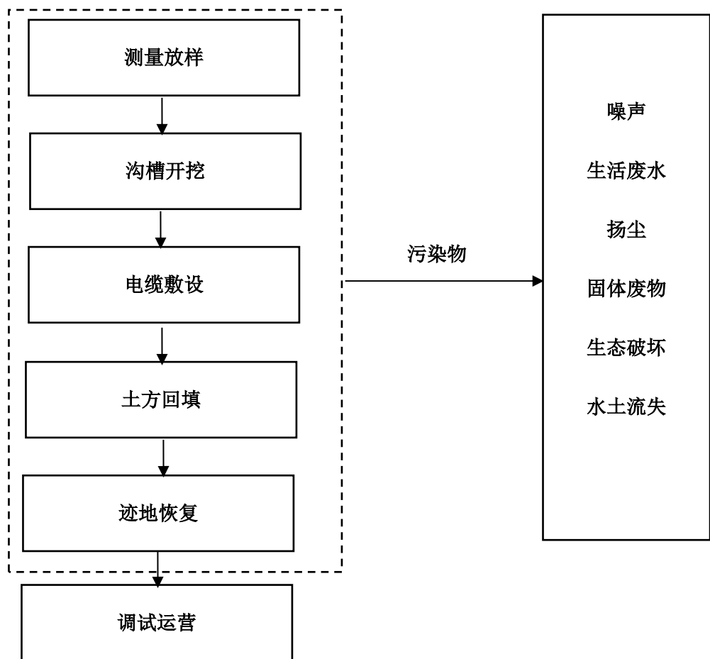
图 4-2 电缆线路施工期主要产污环节示意图
