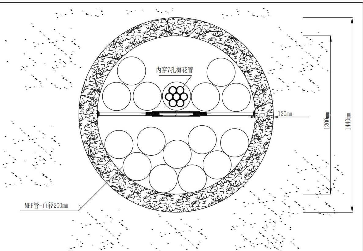
图 2-4 本工程新建电缆顶管示意图
