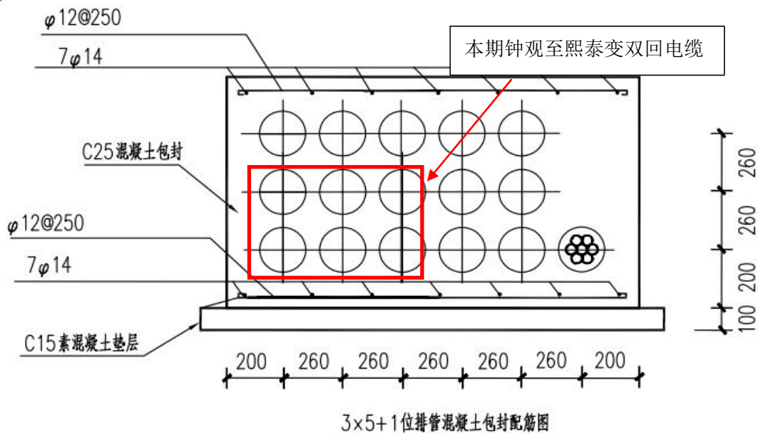
图 2-2 本工程电缆排管示意图
