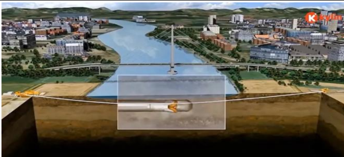
图 2-8 常见拉管施工演示图
