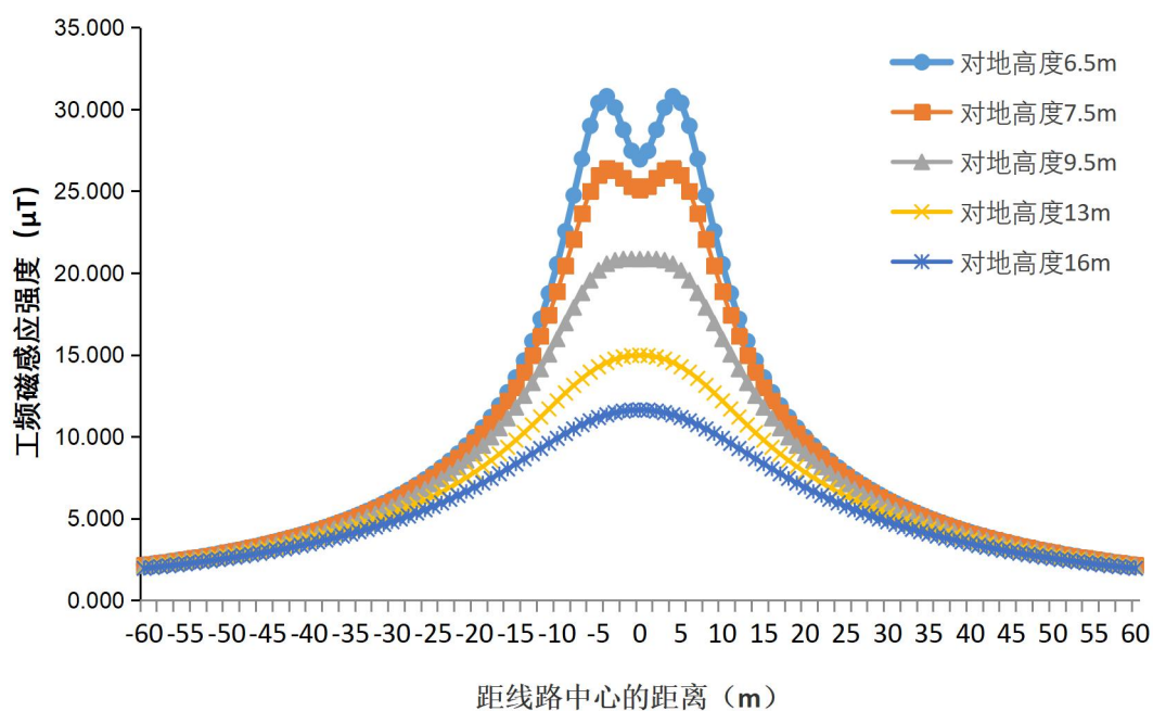
图 3-2 本工程本工程 110/220kV 混压同塔四回架空线路磁感应强度分布趋势图
