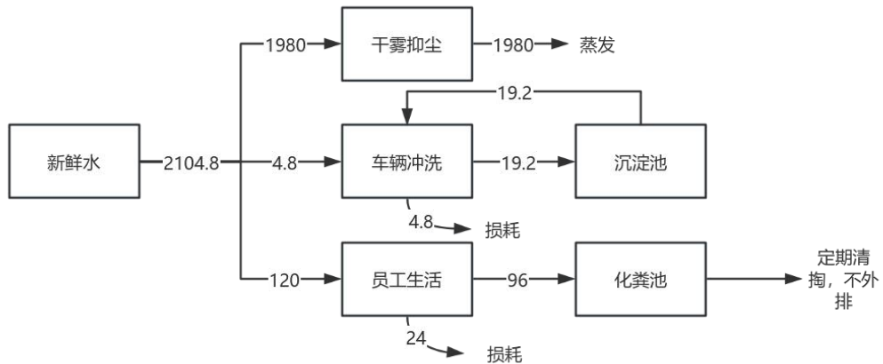
项目水平衡图 (单位: m 3 /a)
