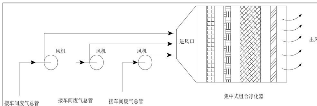
图 4-1 集中式油雾净化工艺示意图
