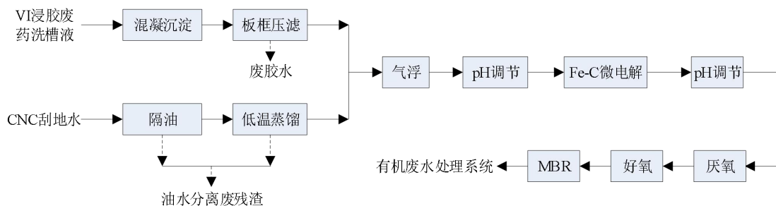
图 4-3 CNC 刮地水、VI 浸胶废药洗槽液处理措施流程图
