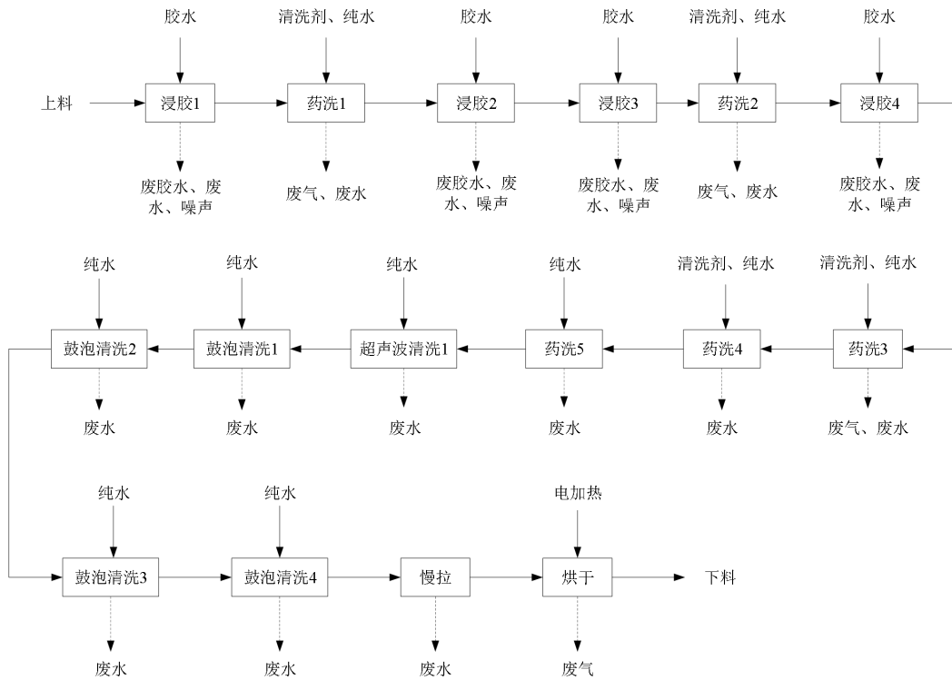
图 2-2 铝件浸胶制程工艺流程及产污环节图
