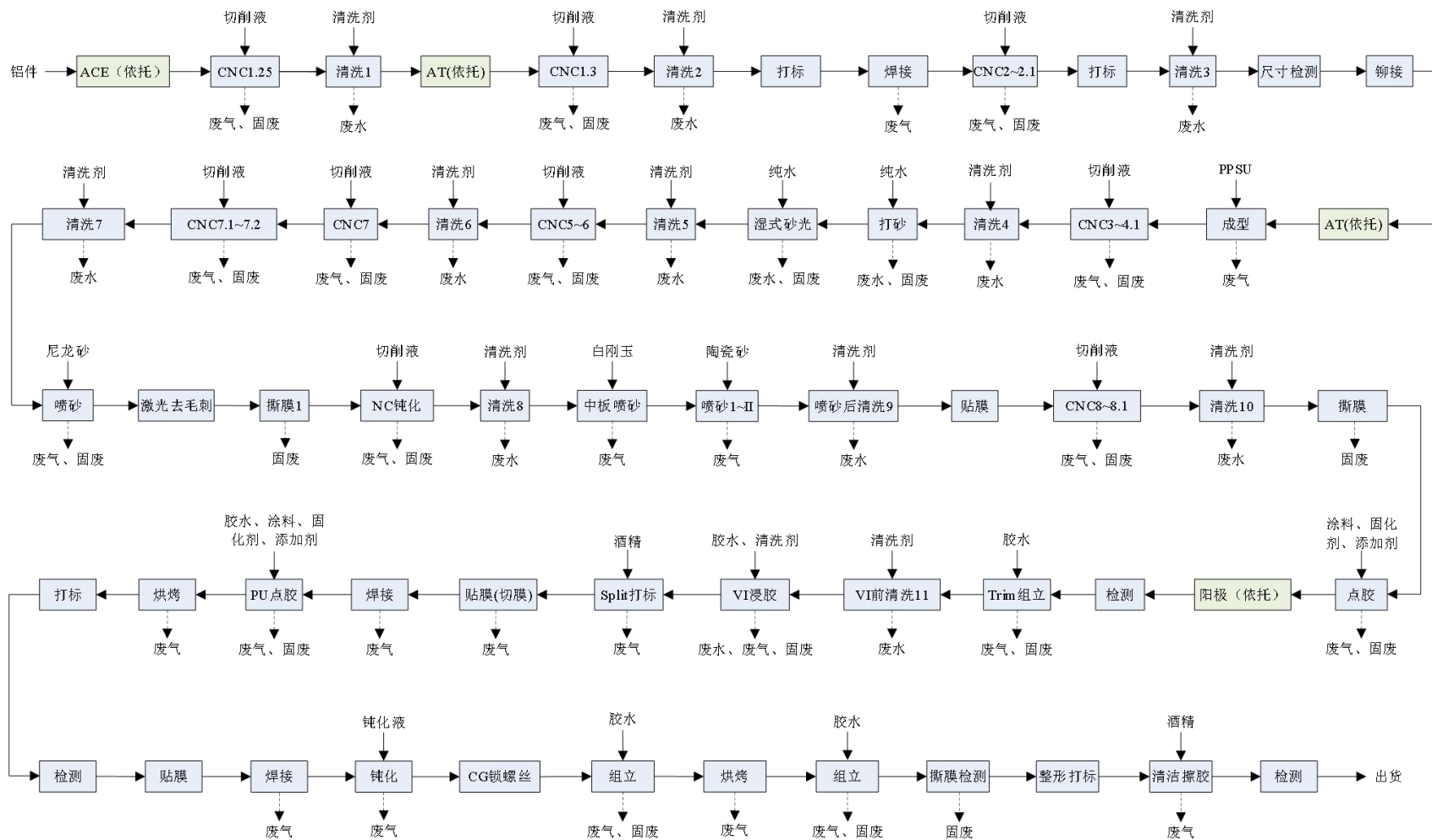
图 2-3 铝件产品工艺流程及产污环节
