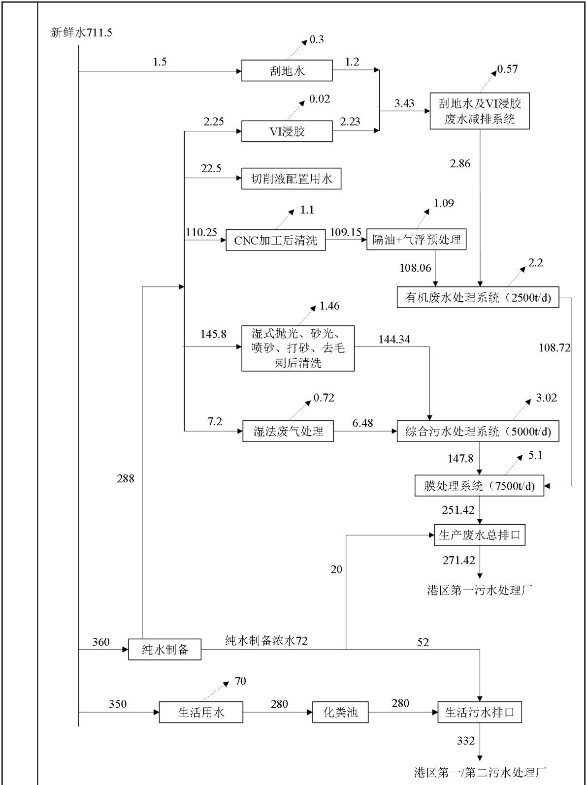
图 2-1 本项目水平衡图 m³/d
