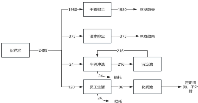
项目水平衡图（单位：m³/a）
