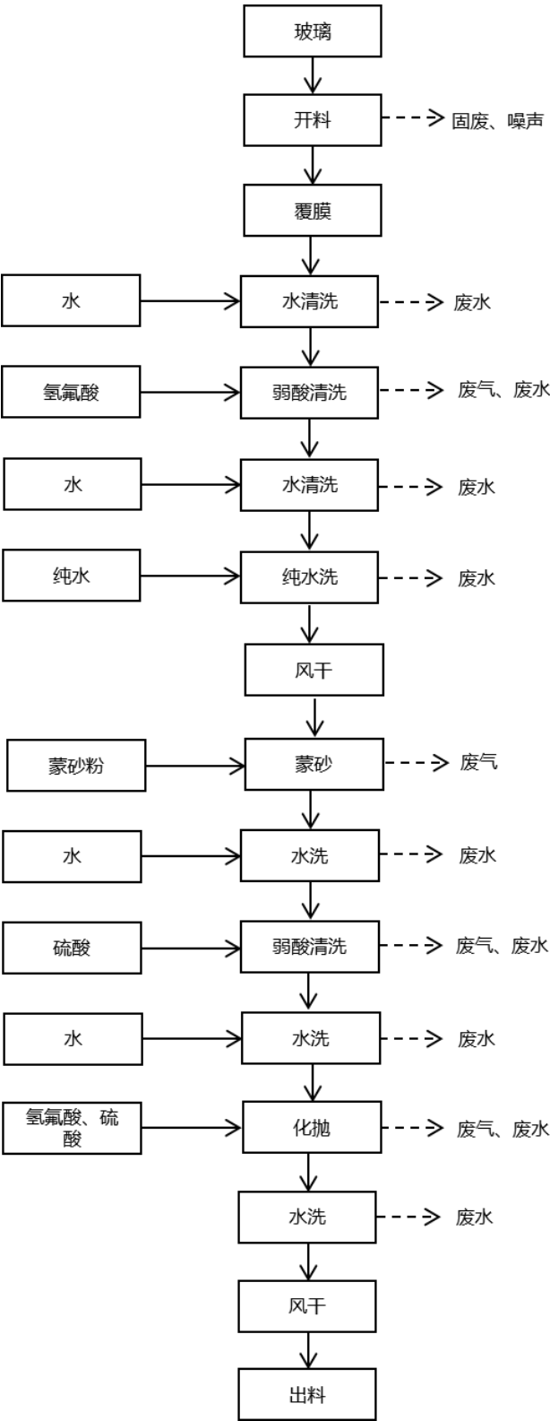
图4. AG玻璃生产工艺及产污环节图
