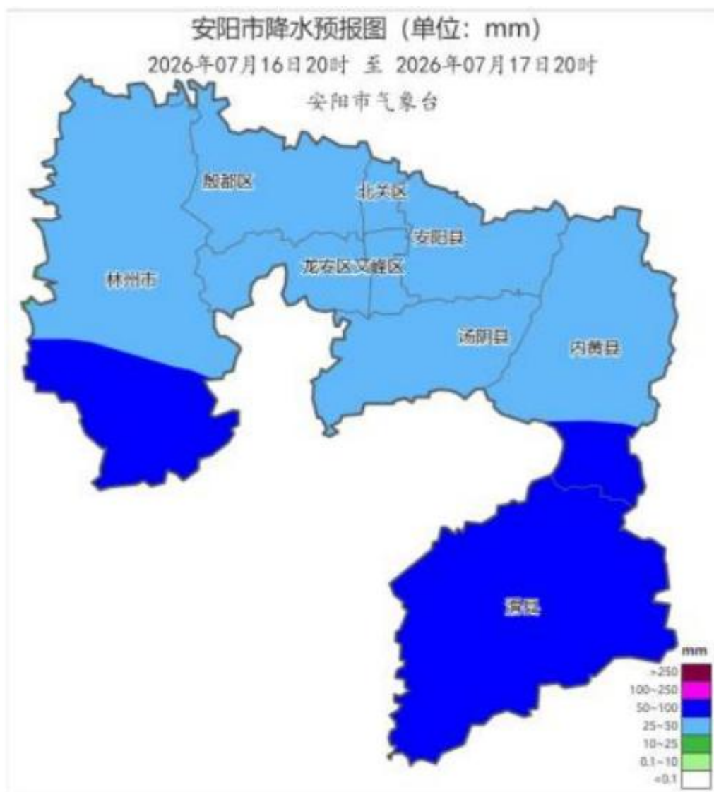
图 1 7 月 16 日 20 时至 17 日 20 时安阳市降水预报图
