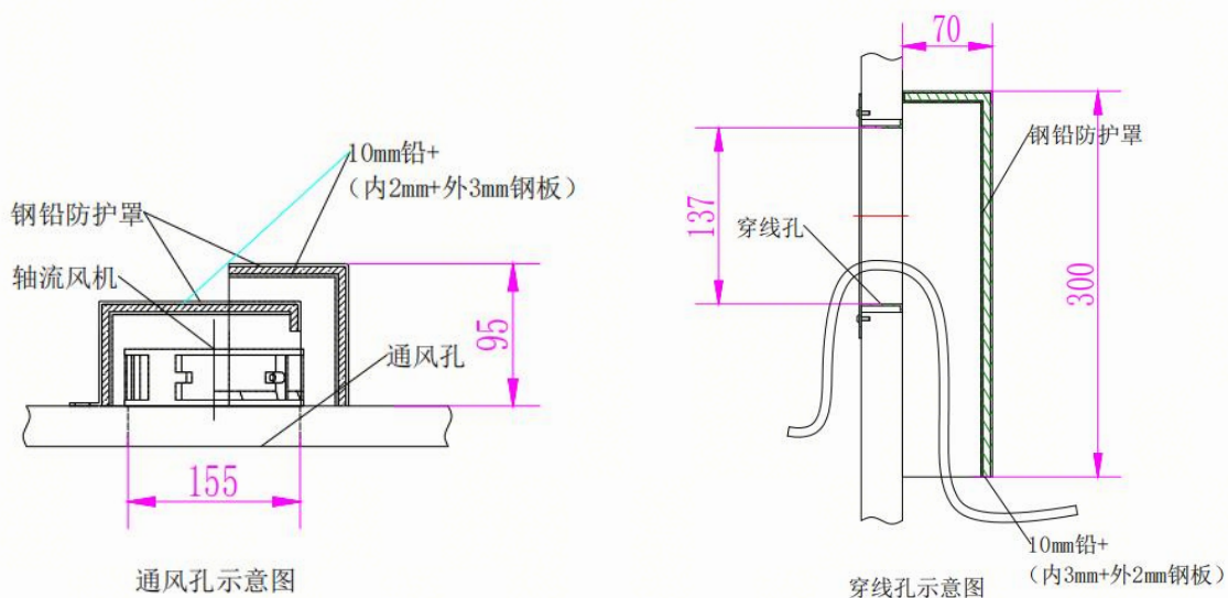
图 10-5 UND225 型 X 射线数字成像检测设备通风孔及穿线孔屏蔽补偿防护示意图
