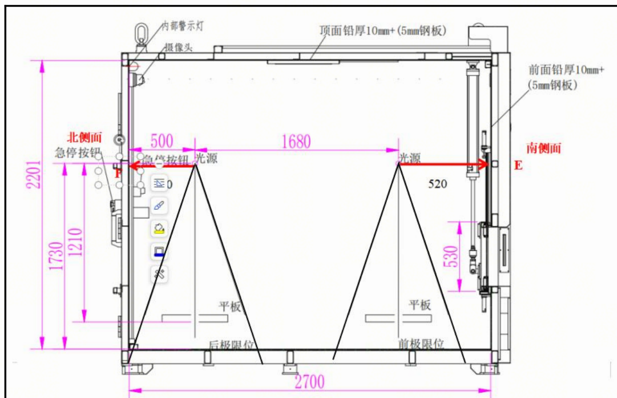
图 11-2 UND225 型 X 射线数字成像检测设备关注点示意图（侧视图）（单位：mm）
