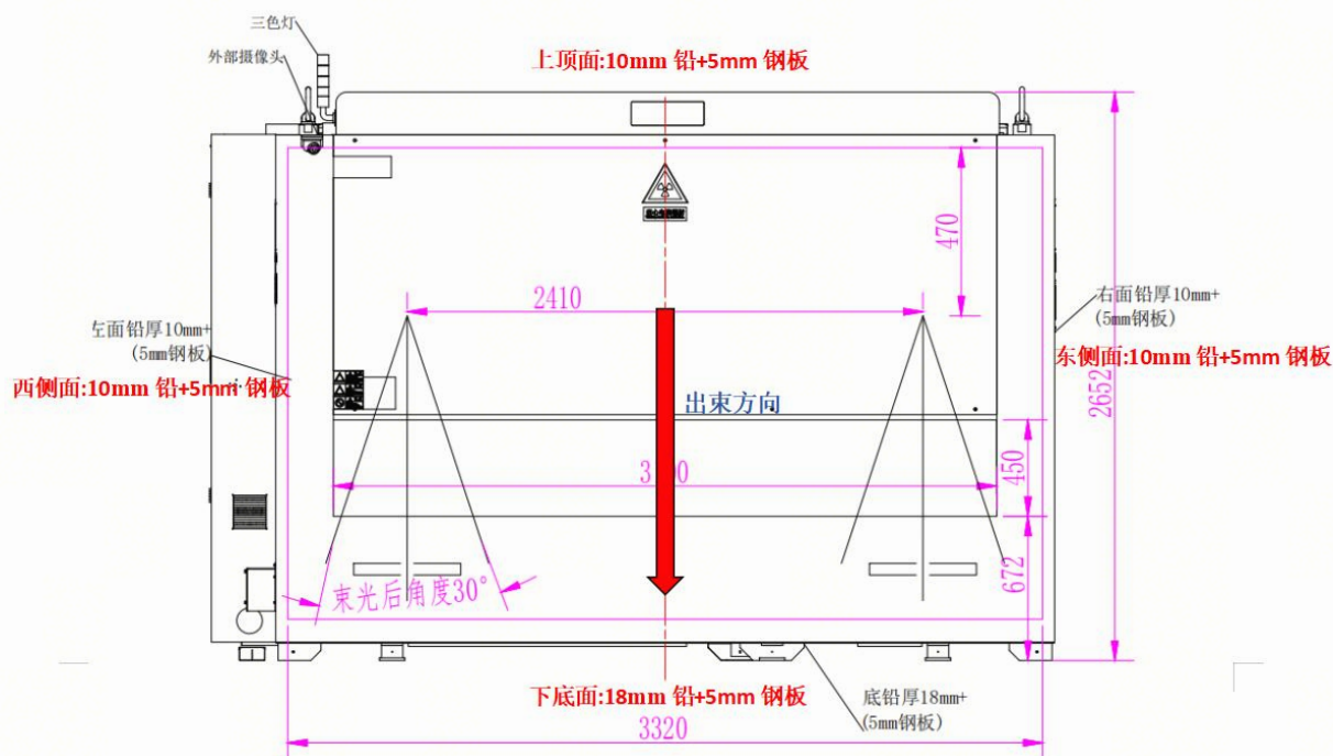
图 10-3 UND225 型 X 射线数字成像检测设备屏蔽防护示意图①
