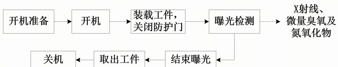
图 9-4 本项目射线装置工作流程
