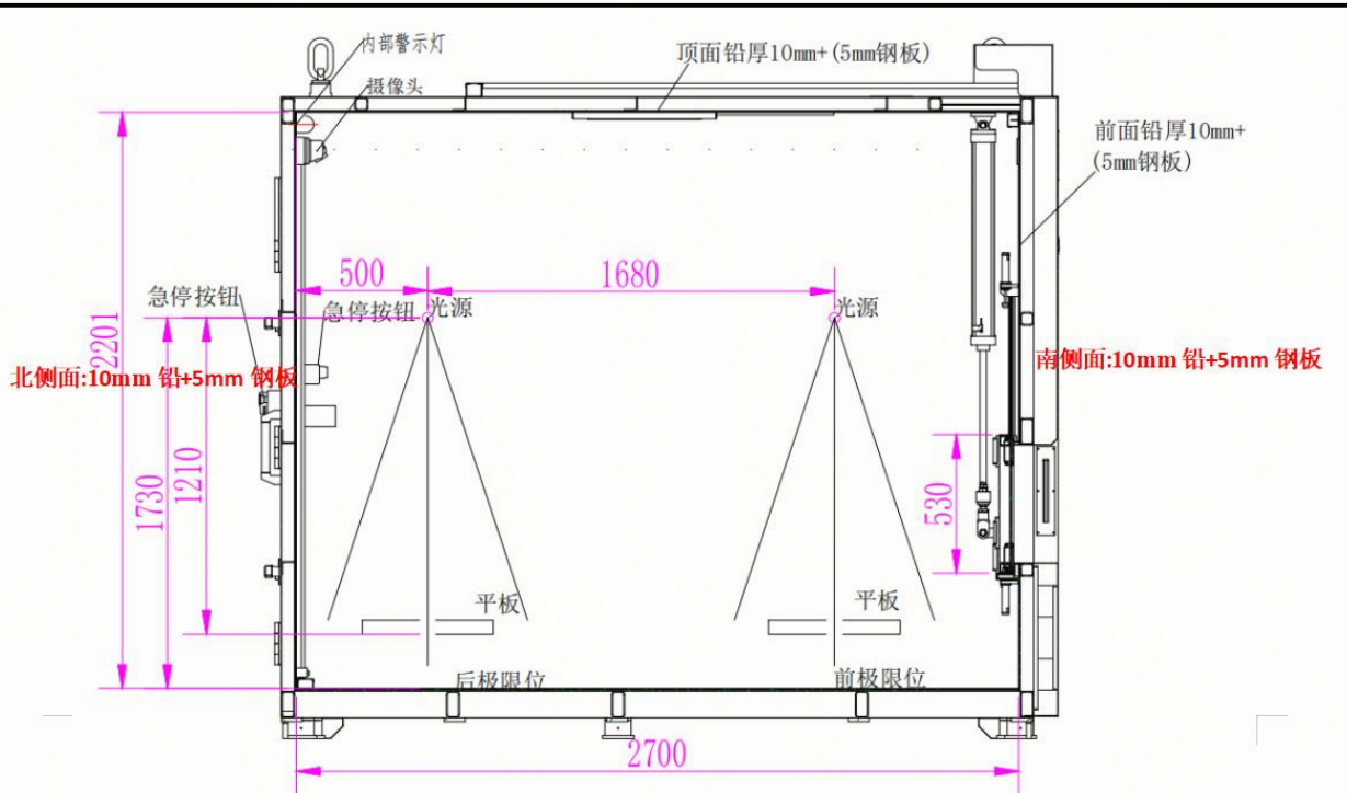
图 10-4 UND225 型 X 射线数字成像检测设备屏蔽防护示意图②
