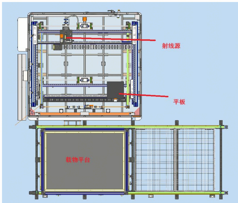
图 9-2 UND225 型 X 射线数字成像检测设备内部结构示意图
