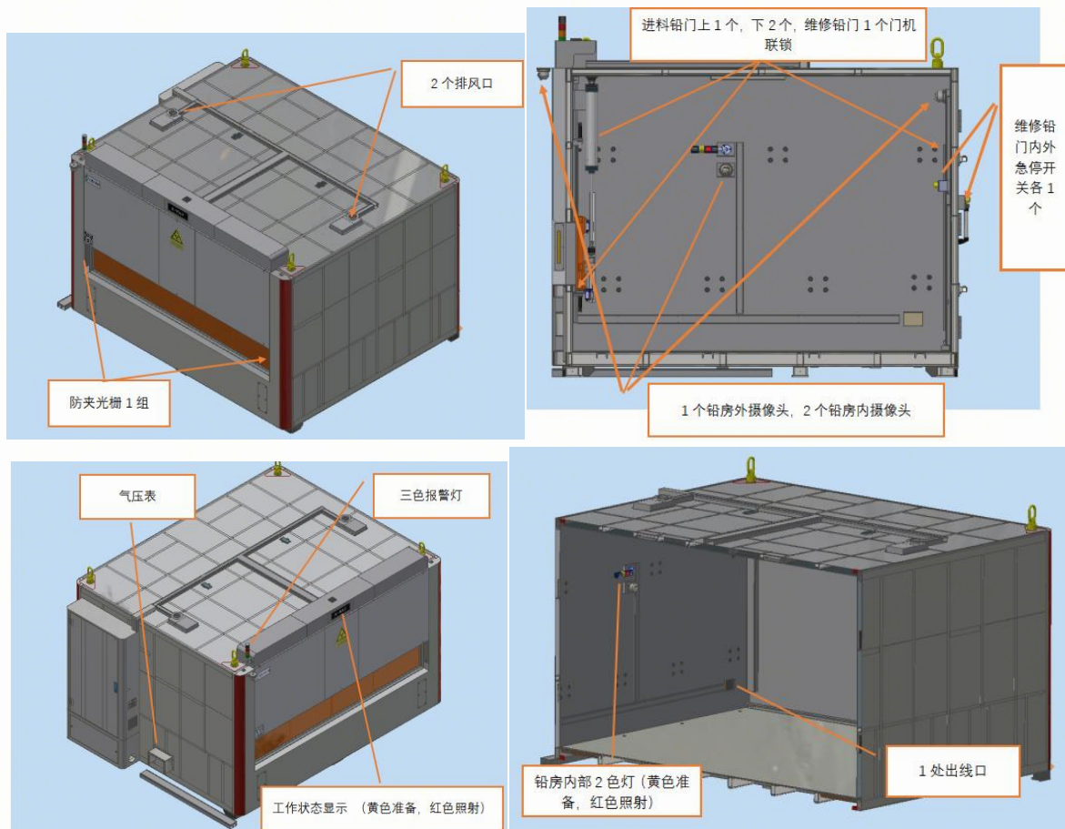
图 10-6 UND225 型 X 射线数字成像检测设备安全设施布局图
