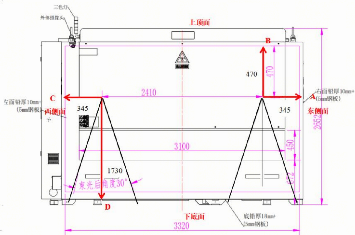
图 11- 1 UND225 型 X 射线数字成像检测设备关注点示意图（正视图）（单位：mm）
