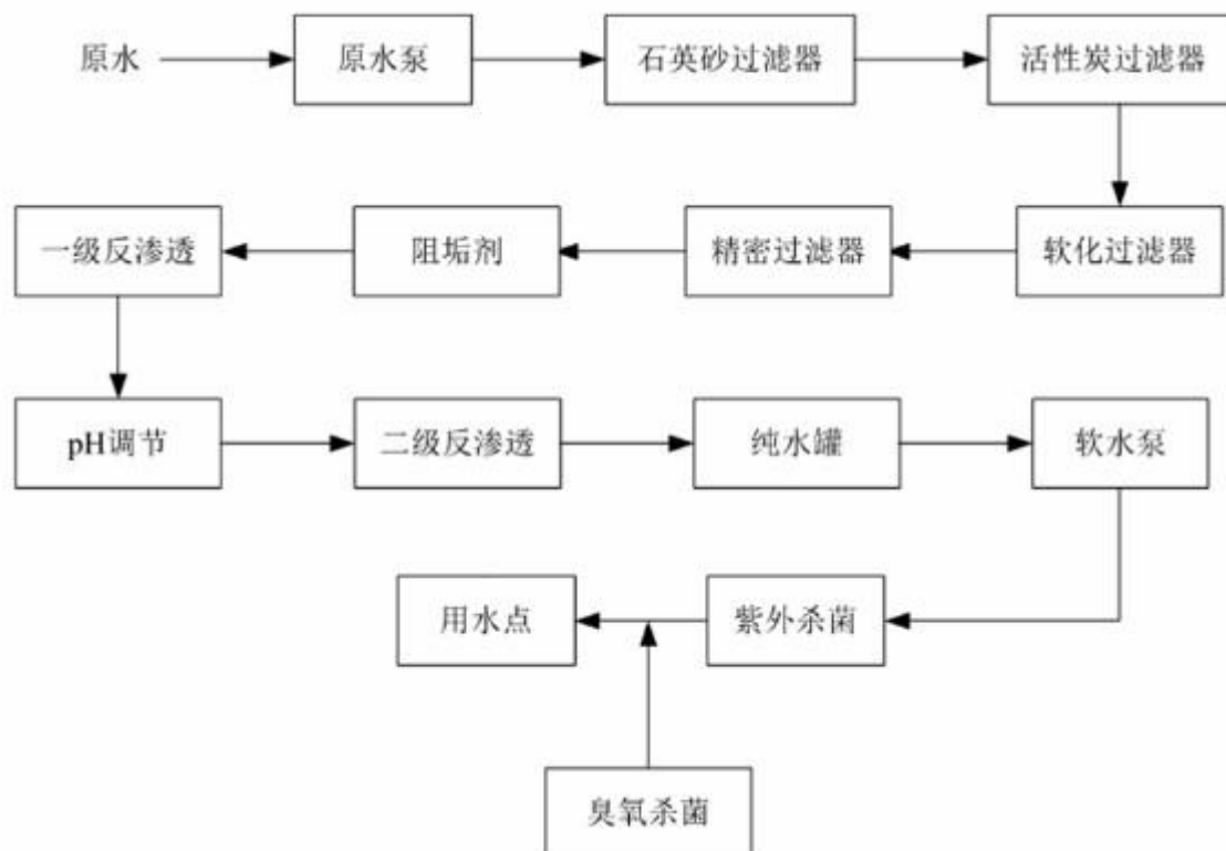
图 7 本项目纯水制备工艺流程图
