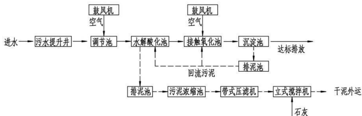
图 8 园区污水处理站工艺流程图
