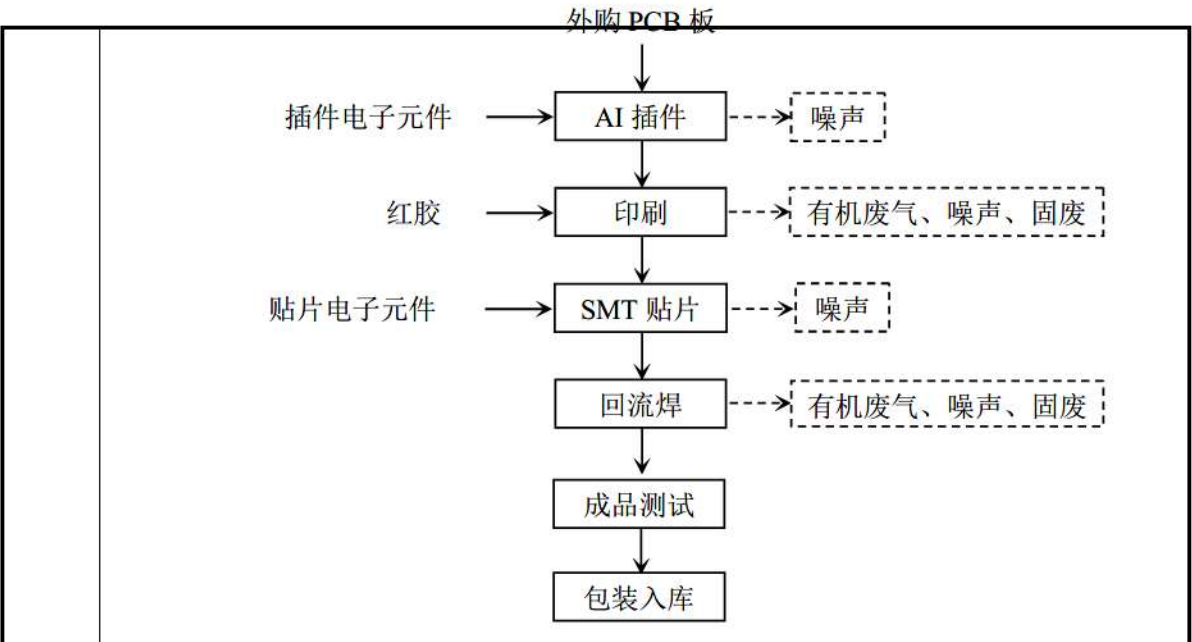
图 2-2 生产工艺及产污环节流程图
