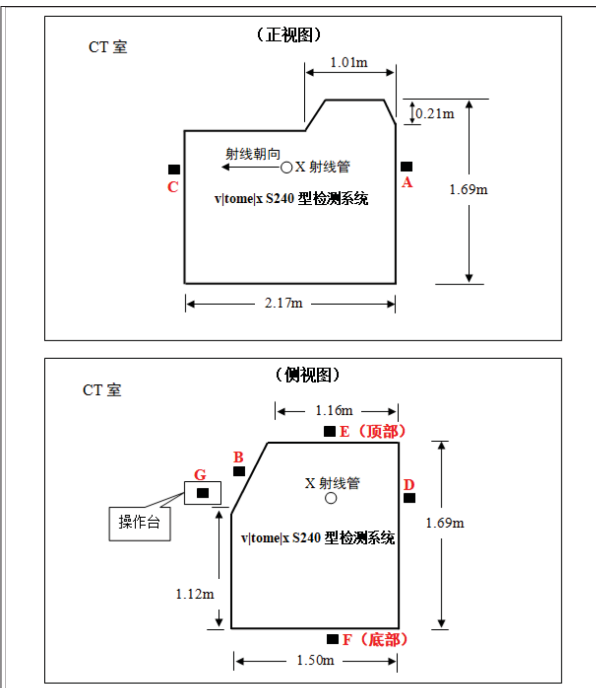
图 11 检测系统各关注点位置示意图
