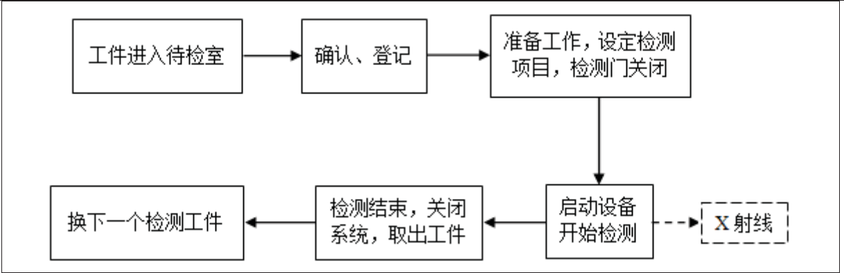
图 9 v|tome|x S240 型 X 射线计算机断层扫描检测系统工作流程图
