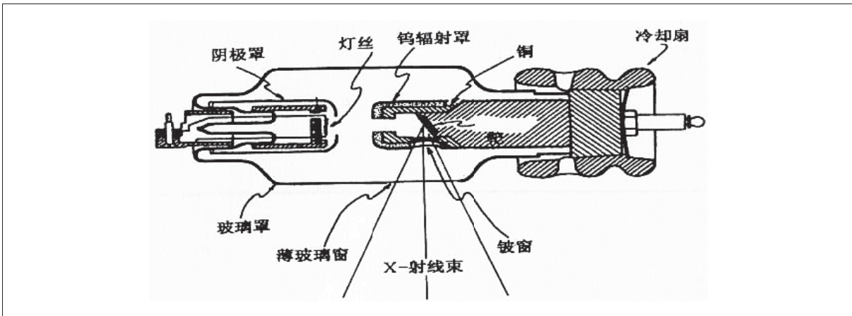
图 7 典型 X 射线管的结构图
