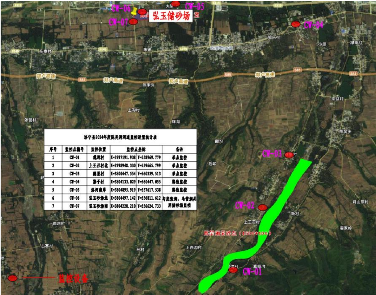
图 3.4-1 洛宁县 2024 年陈吴涧河道采砂监控布置图
