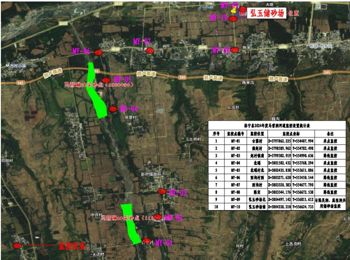
图 3.4-1 洛宁县 2024 年马营涧河道采砂监控布置图
