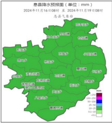
图 1 2024 年 11 月 16 日 08 时-19 日 08 时息县降水预报图
