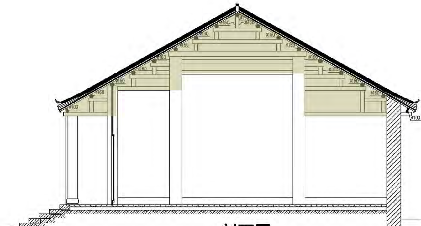
剖面图
