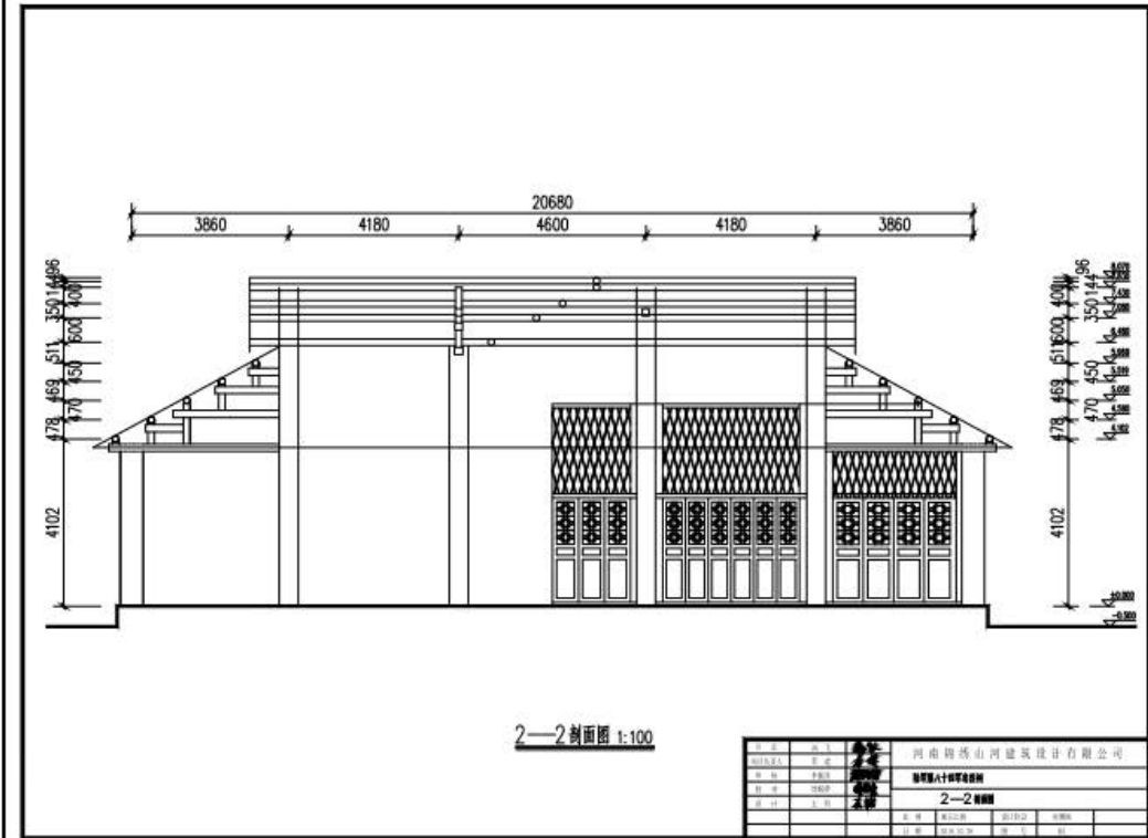
忠烈祠剖面图 5
