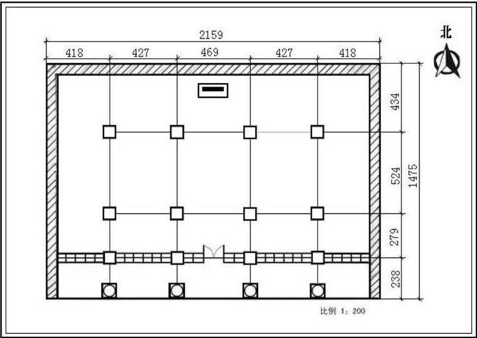
陆军第八十四军忠烈祠平面示意图 比例 1:200
