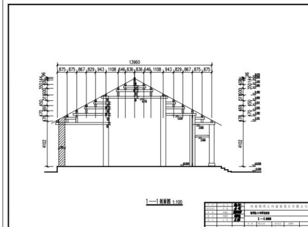
忠烈祠剖面图 4
