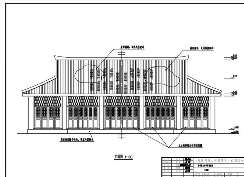
忠烈祠立面图 3
