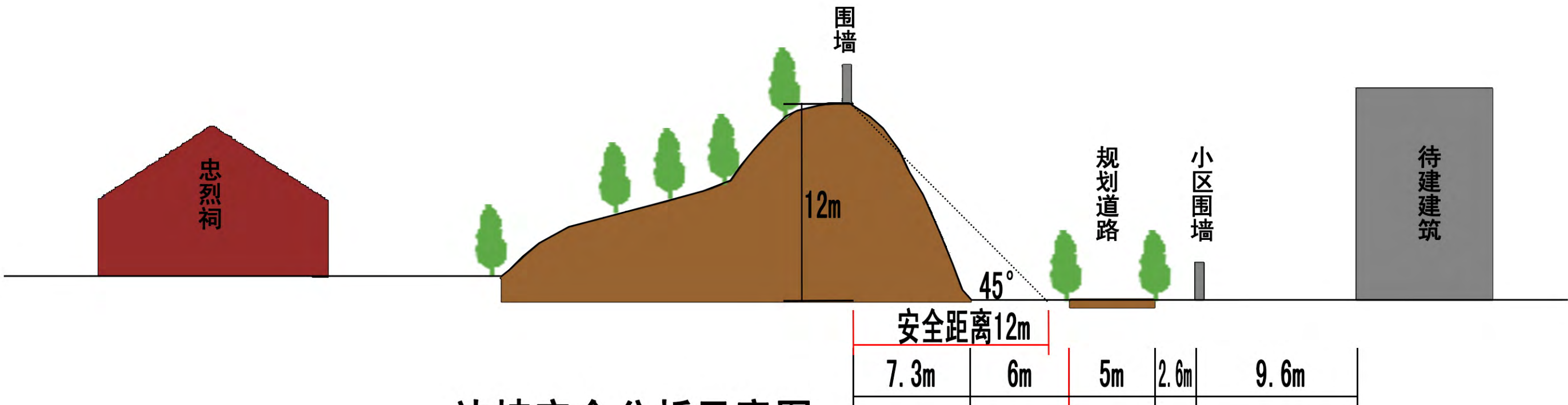
边坡安全分析示意图
