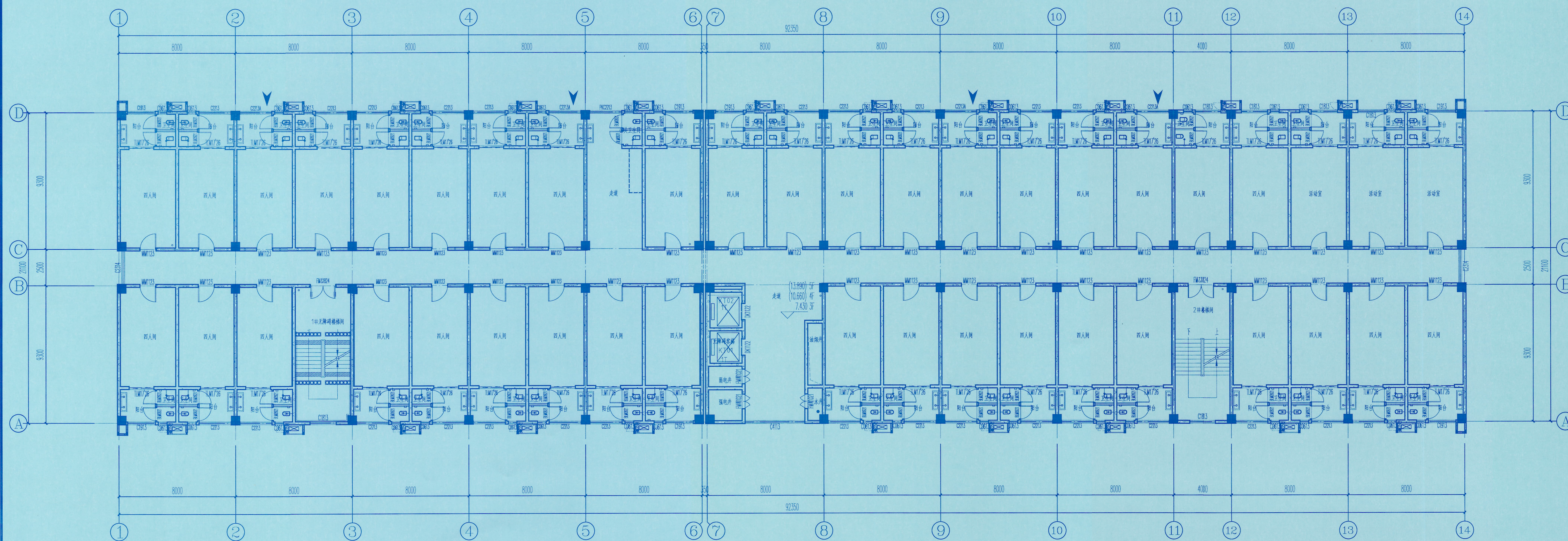
三 五层平面图 1:150
