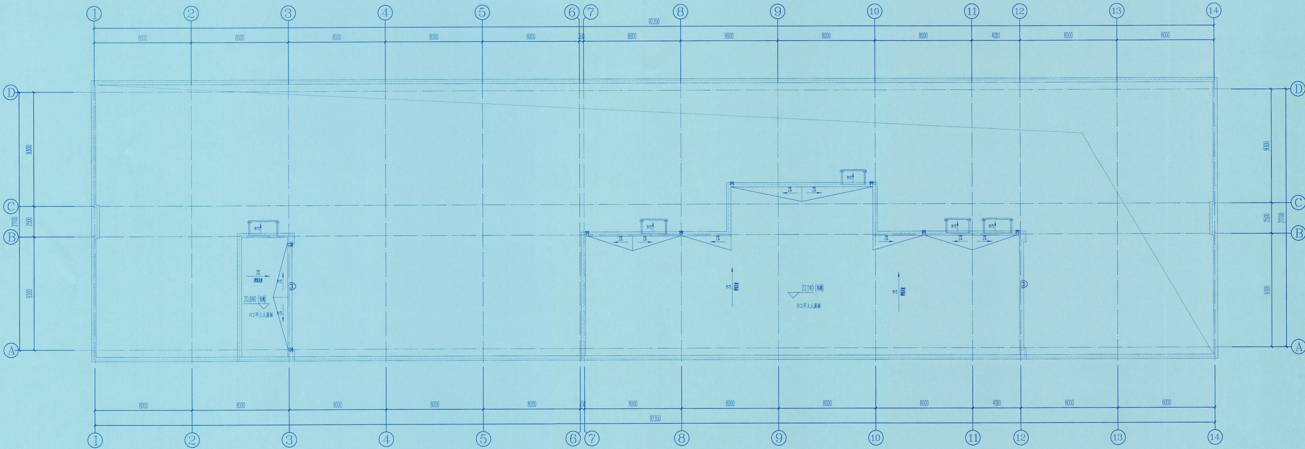
构架层平面图 1:150
